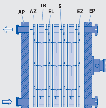
预涂过滤机的结构示意图：
